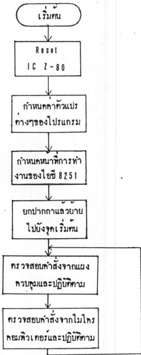
รูปที่ ๔.๑ ผังการทำงานเมื่อเริ่มเปิดเครื่องพลอทเตอร์
