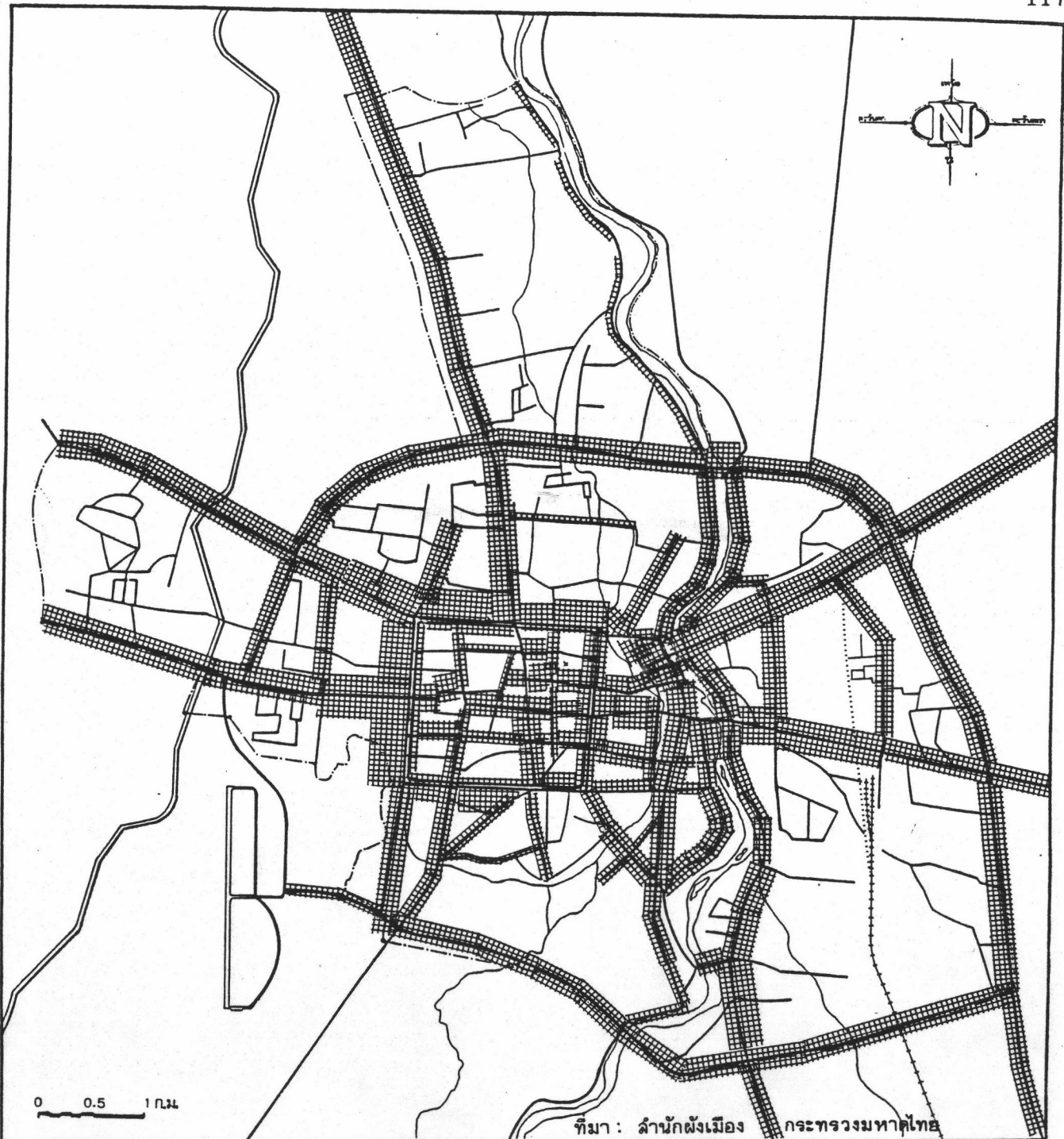
แผนที่ 3.22 แสดง ปริมาณการจราจรในช่วงโมงเร่งด่วน พ.ศ. 2531
