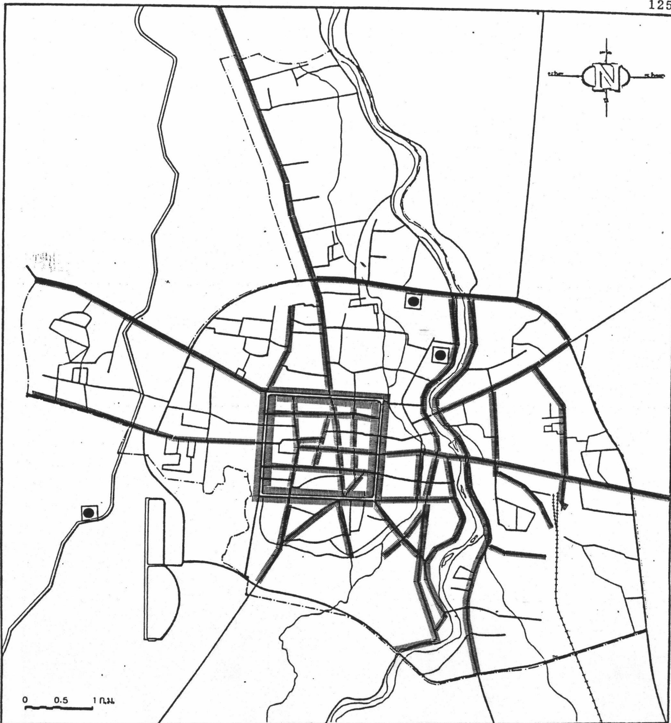
แผนที่ 3.23 แสดง ตำแหน่งโรงกรองน้ำและแนวท่อประปา
