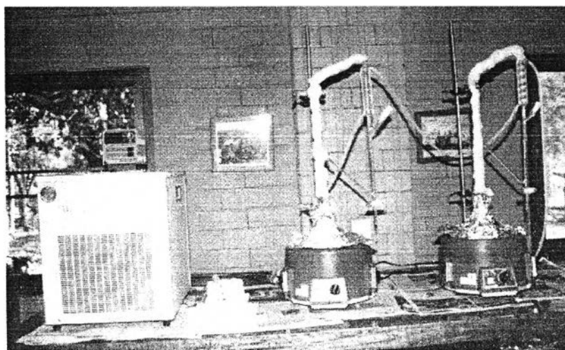
เครื่องกลั่นน้ำมันหอมระเหย ที่นำมาทดสอบหาปริมาณ น้ำมันยูคาลิปตัส ที่มีสาย พันธ์แตกต่างกัน
