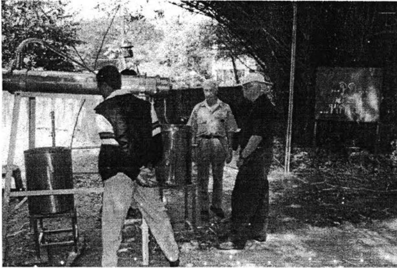
ทดลองกลั่นน้ำมัน ด้วย เครื่องกลั่นขนาดใหญ่ ที่ได้รับการสนับสนุน จากออสเตรเลีย
