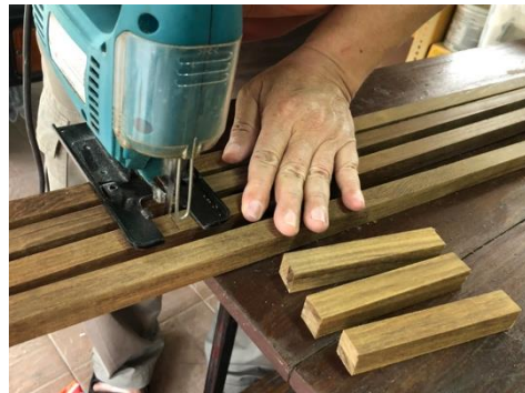
ภาพที่ 304 เลื่อยแป้นกด ที่มา : ผู้วิจัย
