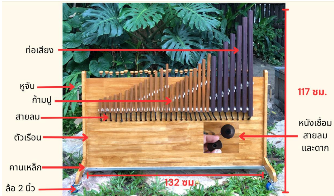
ภาพที่ 52 สัดส่วนและส่วนประกอบลมรายด้านหน้าที่พัฒนา ครั้งที่ 2
