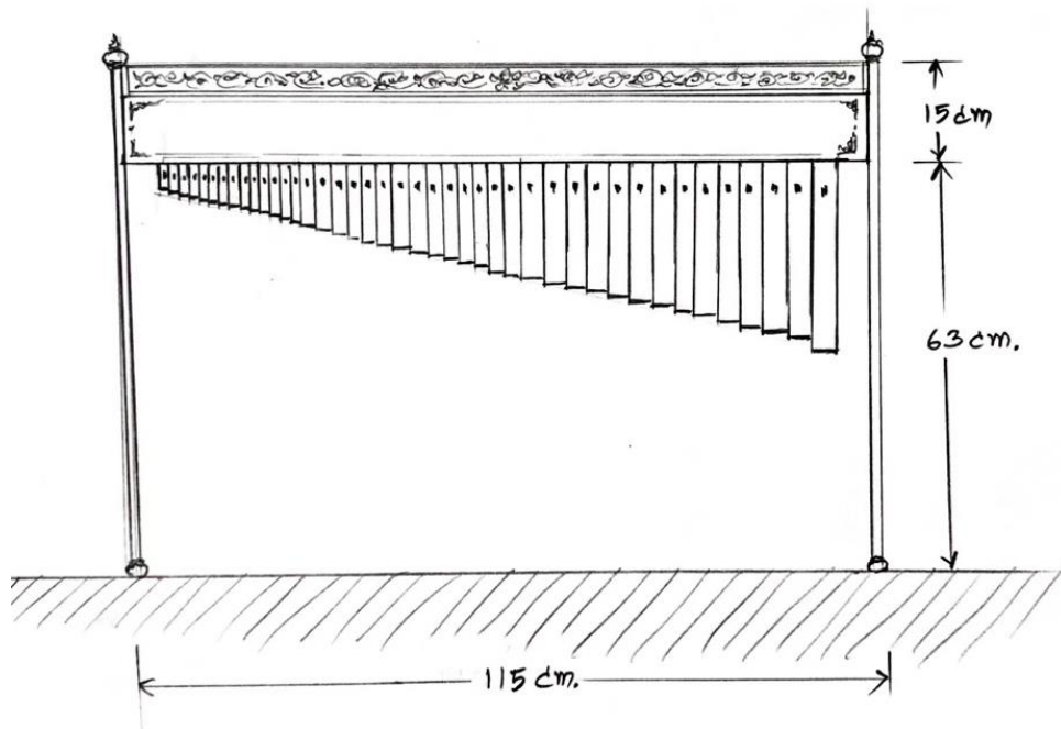
ภาพที่ 36 แบบร่างลมรายครั้งที่ 1 มุมมองด้านหน้า ที่มา : วิรัช สงเคราะห์
