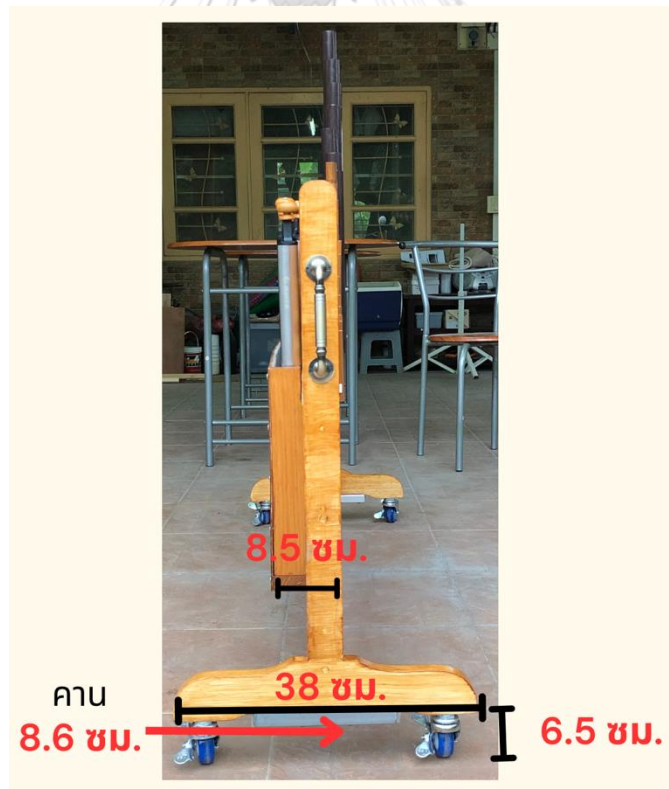
ภาพที่ 54 สัดส่วนและส่วนประกอบระบบลมภายในของลมรายที่พัฒนา ครั้งที่ 2 ที่มา : ผู้วิจัย
