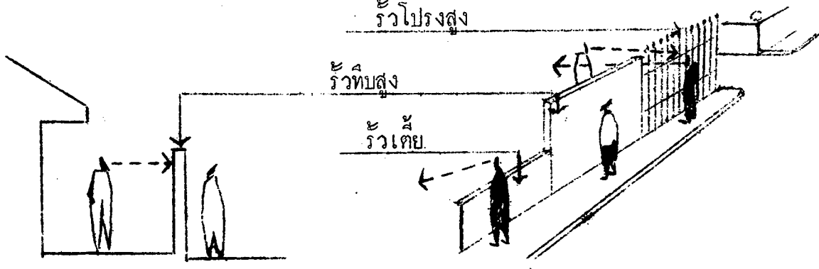
รูปที่ 17 ความทึบ - โปร่งของรั้วบ้านกับการมองเห็น
