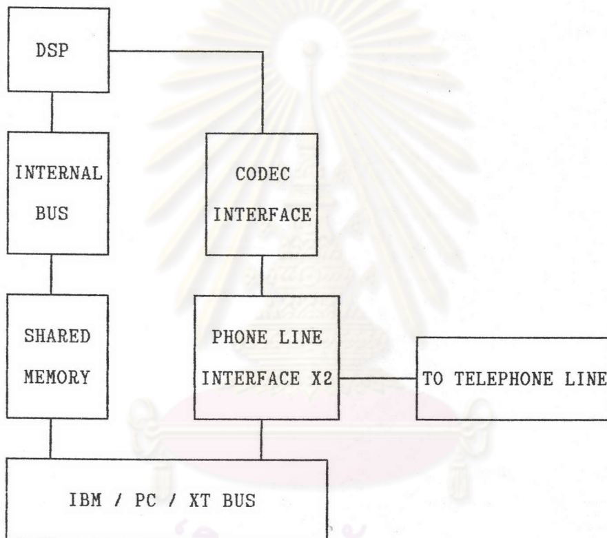
รูปที่ จ.1 แบบการทำงานของแผงวงจรเสียง
