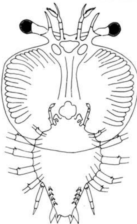
รูป 29 แสดง Larval stage VI-VIII ของ Scyllarides sp.
