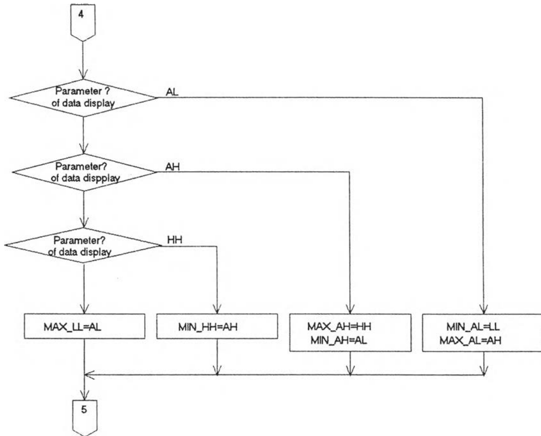
รูปที่ 4.4 แสดงผังงานของโปรแกรมการบริการปุ่มกด (ต่อ)
