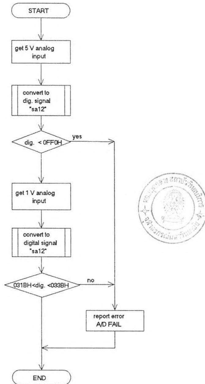
รูปที่ 4.10 แสดงผังงานของการทำงานของโปรแกรมการตรวจสอบอินพุตเกินพิสัย
