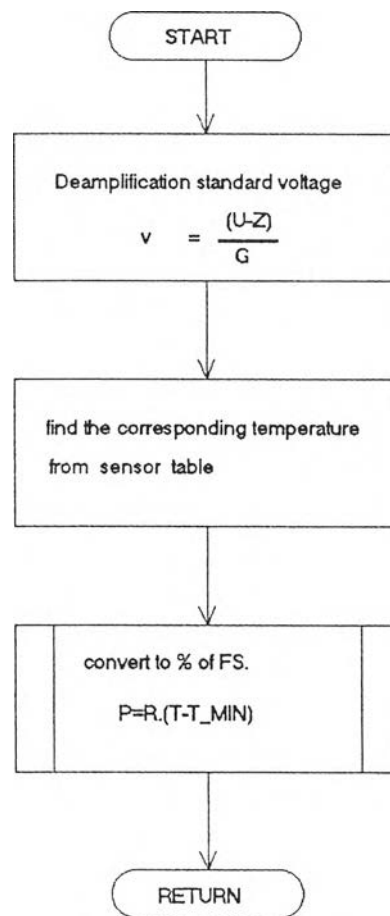
รูปที่ 4.14 แสดงผังงานของโปรแกรม Linear_and_convert
