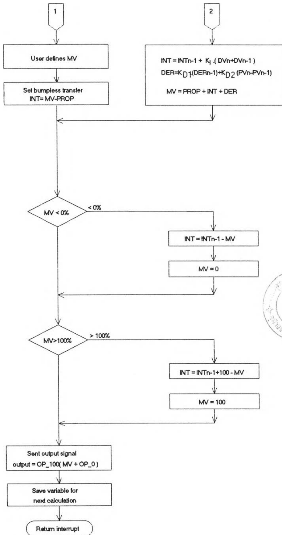
รูปที่ 4.1 ข) แสดงผังงานของการคำนวณการควบคุมแบบ PID (ต่อ)
