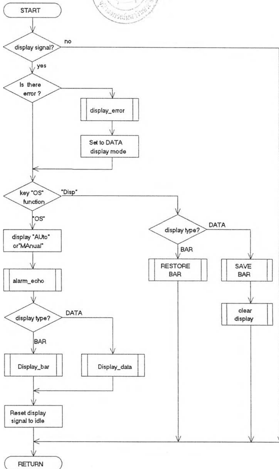
รูปที่ 4.5 แสดงผังงานของโปรแกรมการแสดงผล
