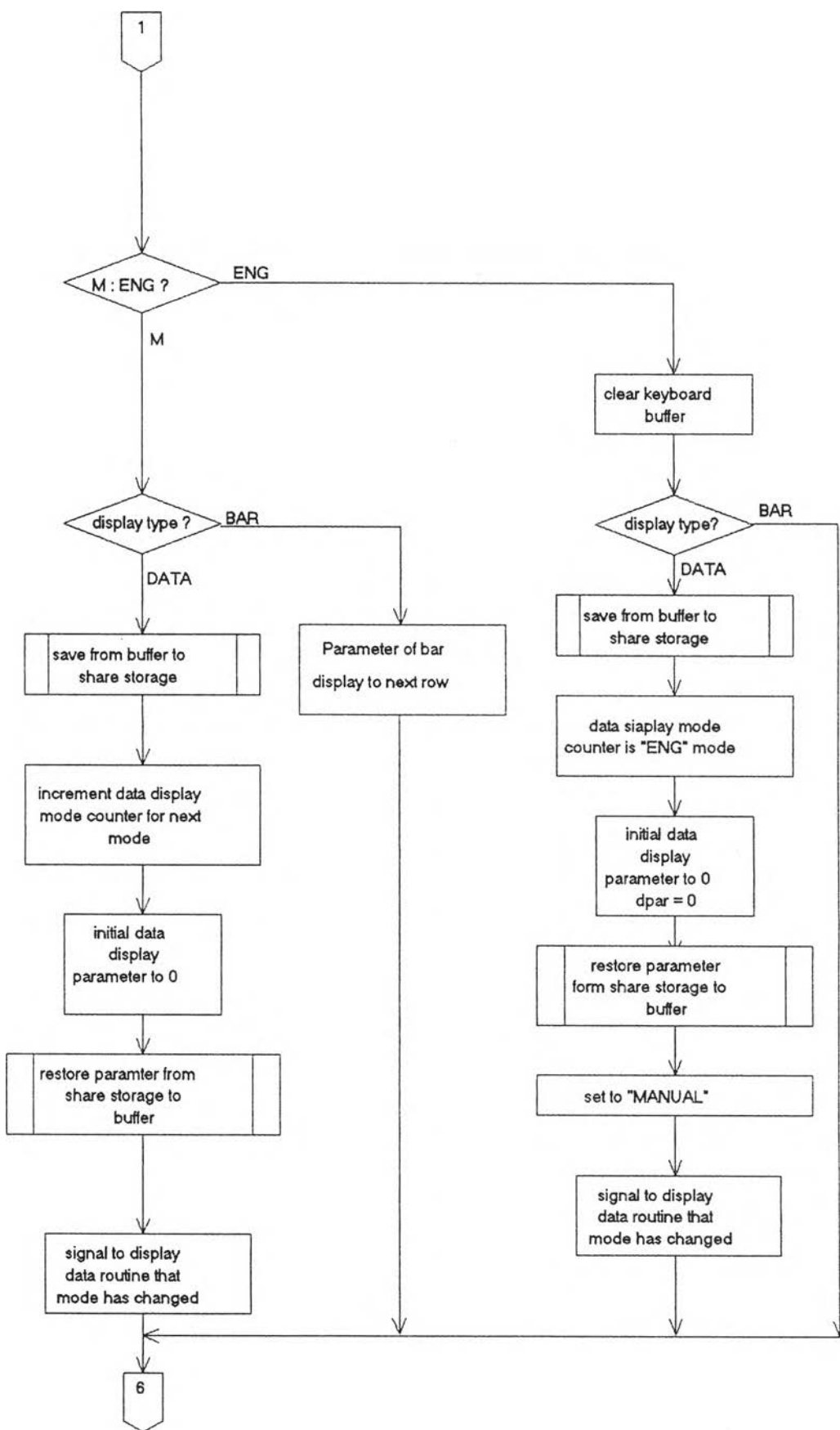
รูปที่ 4.4 แสดงผังงานของโปรแกรมการบริการปุ่มกด (ต่อ)
