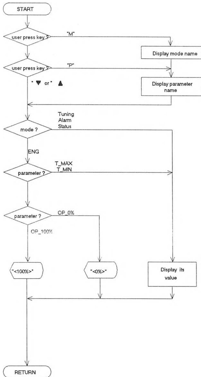
รูปที่ 4.6 แสดงผังงานการทำงานของส่วนแสดงผลแบบแสดงค่าข้อมูล
