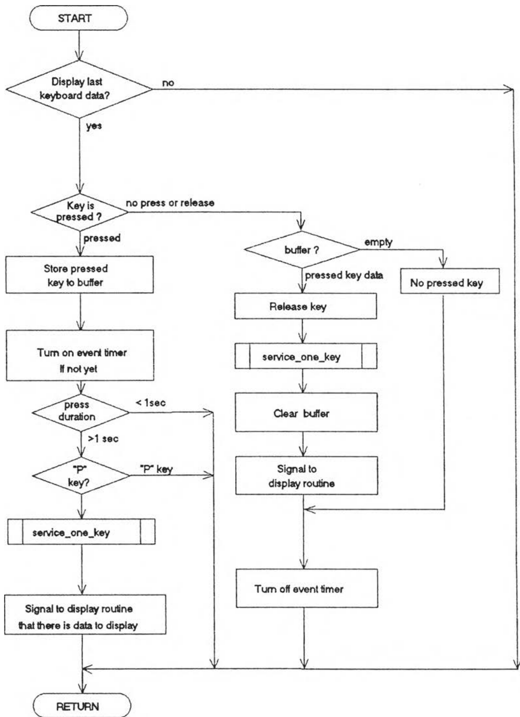
รูปที่ 4.3 แสดงผังงานของส่วนการรับข้อมูลจากปุ่มกด
