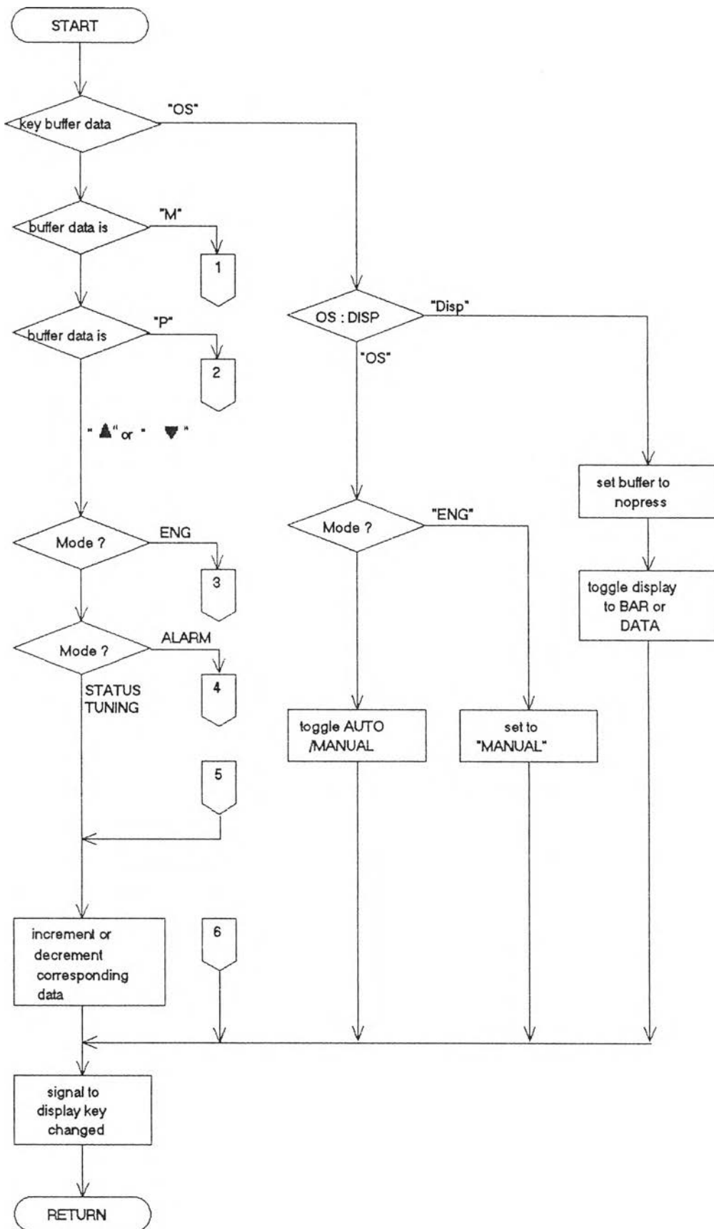
รูปที่ 4.4 แสดงผังงานของโปรแกรมการบริการปุ่มกด
