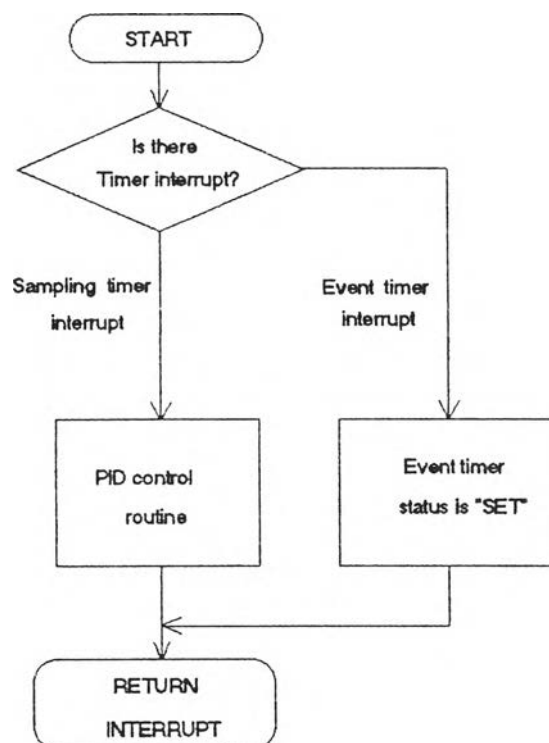
รูปที่ 4.1 ก) แสดงผังงานของโปรแกรมอินเทอร์รัพต์
