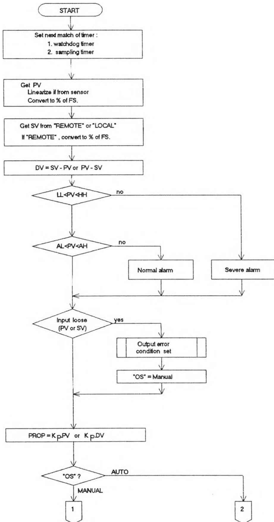
รูปที่ 4.1 ข) แสดงผังงานของการคำนวณการควบคุมแบบ PID (PID control routine)
