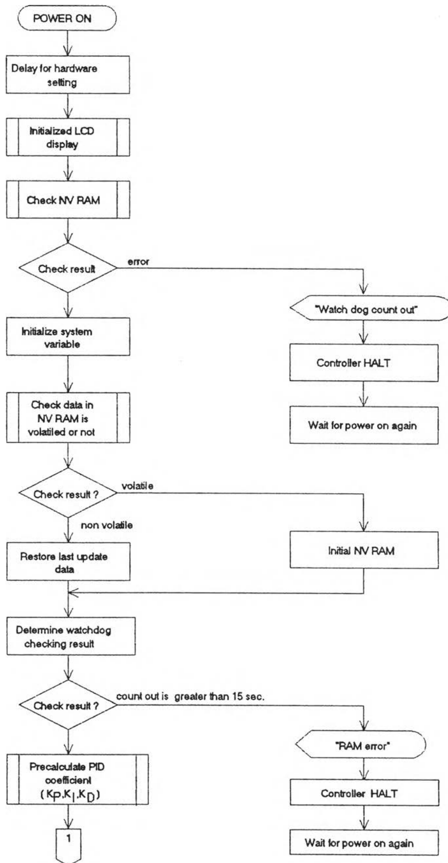
รูปที่ 4.2 แสดงผังงานของโปรแกรมหลัก
