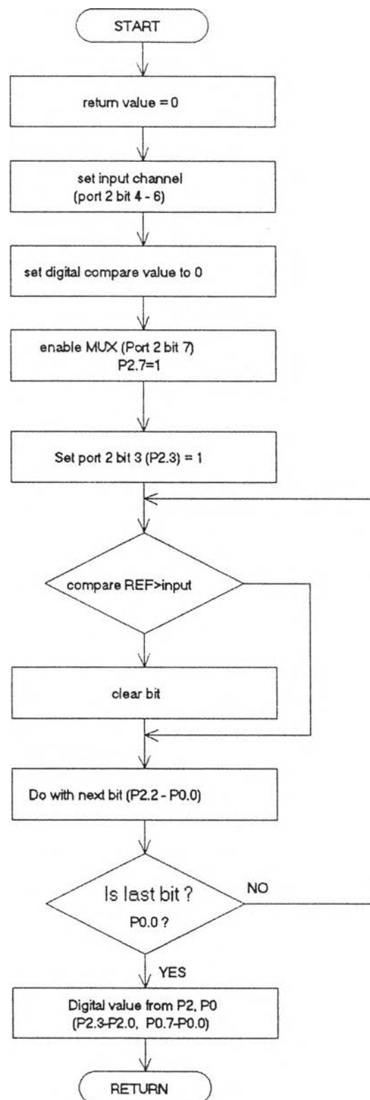
รูปที่ 4.11 แสดงผังงานของโปรแกรมการประมาณค่าอินพุตแบบ Successive
