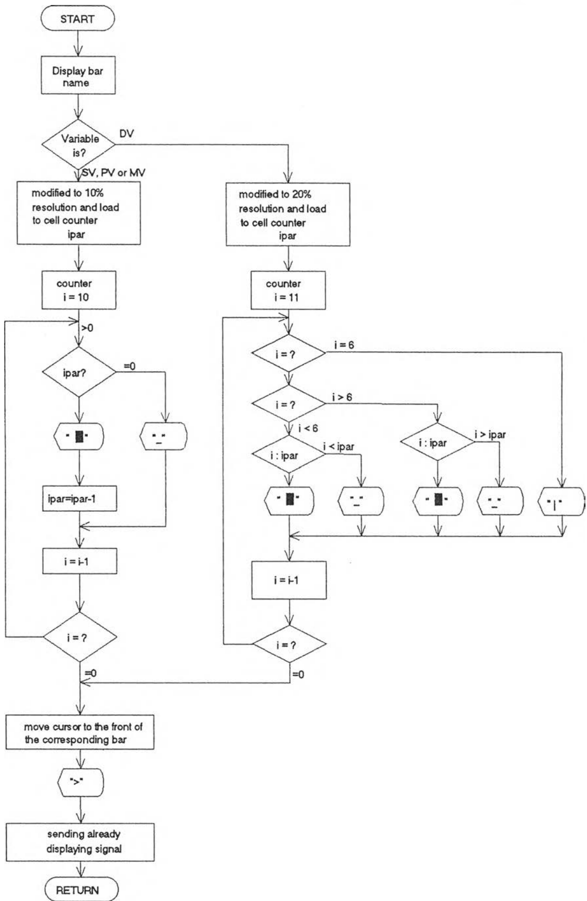
รูปที่ 4.7 แสดงผังงานการทำงานของส่วนแสดงผลแบบกราฟแท่ง
