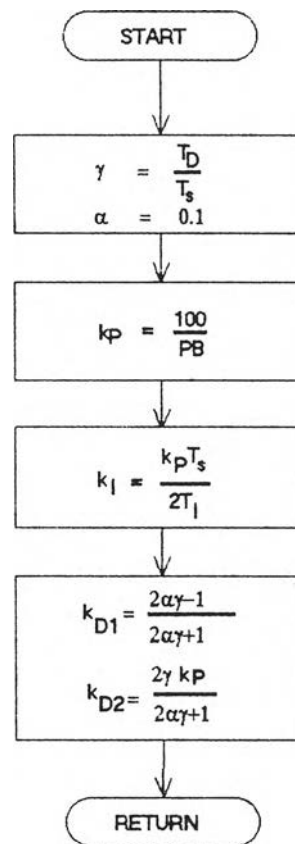
รูปที่ 4.15 แสดงผังงานของการคำนวณสัมประสิทธิ์ของ PID
