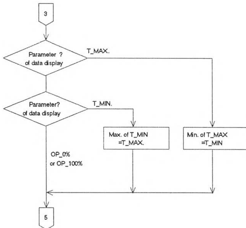
รูปที่ 4.4 แสดงผังงานของโปรแกรมการบริการปุ่มกด (ต่อ)
