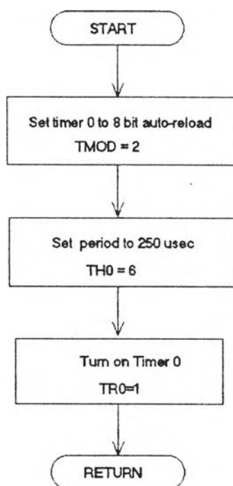
รูปที่ 4.16 โปรแกรมการกำหนดค่าฐานเวลาสำหรับมอดูล PCA "Init_timebase"
