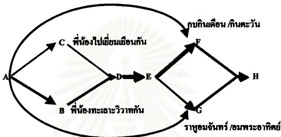
ภาพ : แสดงสูตรโครงสร้าง (syntax) ของตำนานสุริยคราสและจันทรคราสของชนชาติไท
